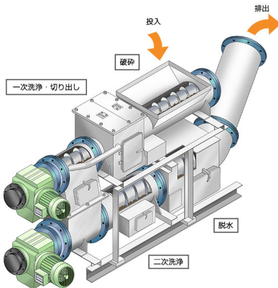
構造概念図
