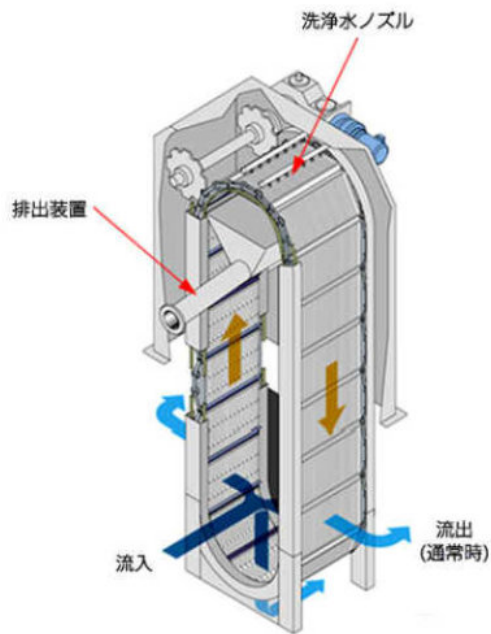
構造概念図
