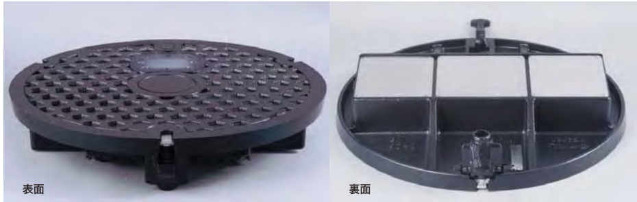
図-2 マンホールアンテナ外観写真
